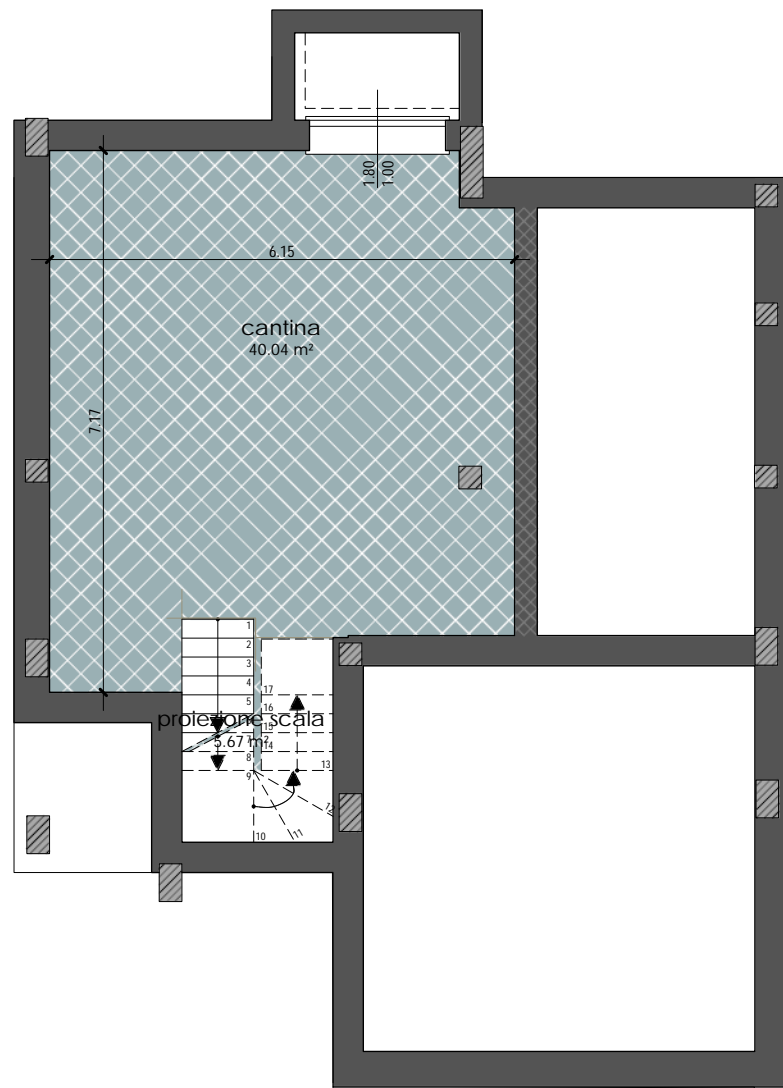
Piano Interrato - Lotto 2 Scala 1:100
