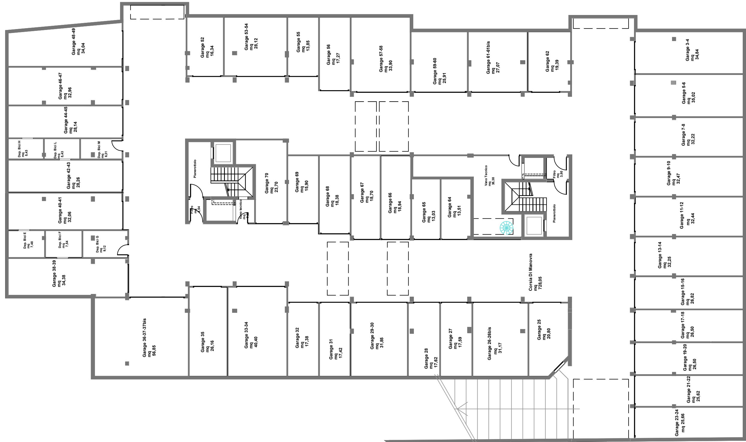
INTERRATO SCALA 1:200
