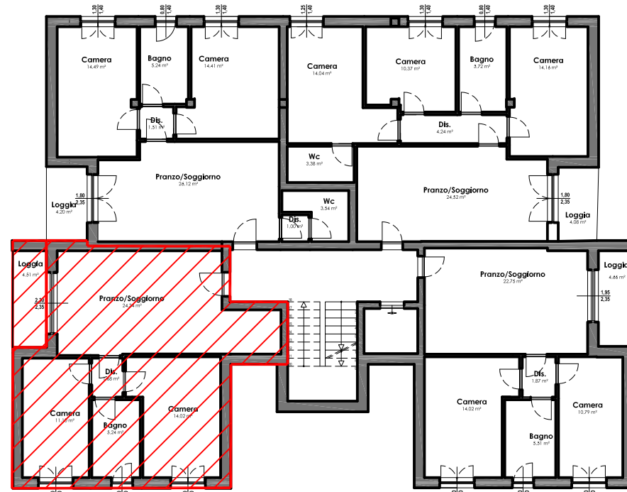
INQUADRAMENTO SCALA 1:200
