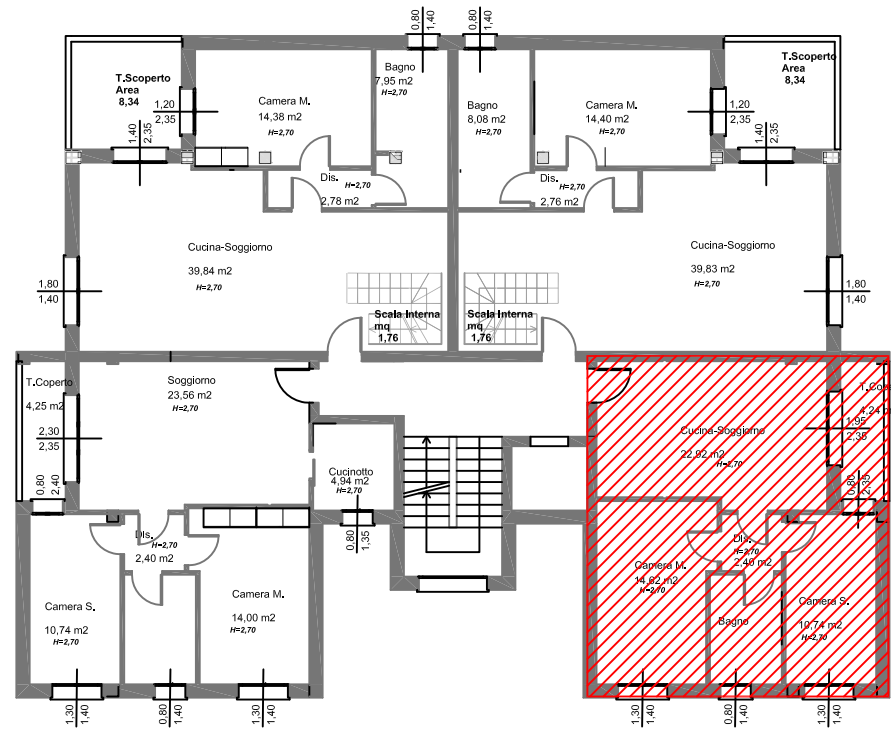
INQUADRAMENTO SCALA 1:200
