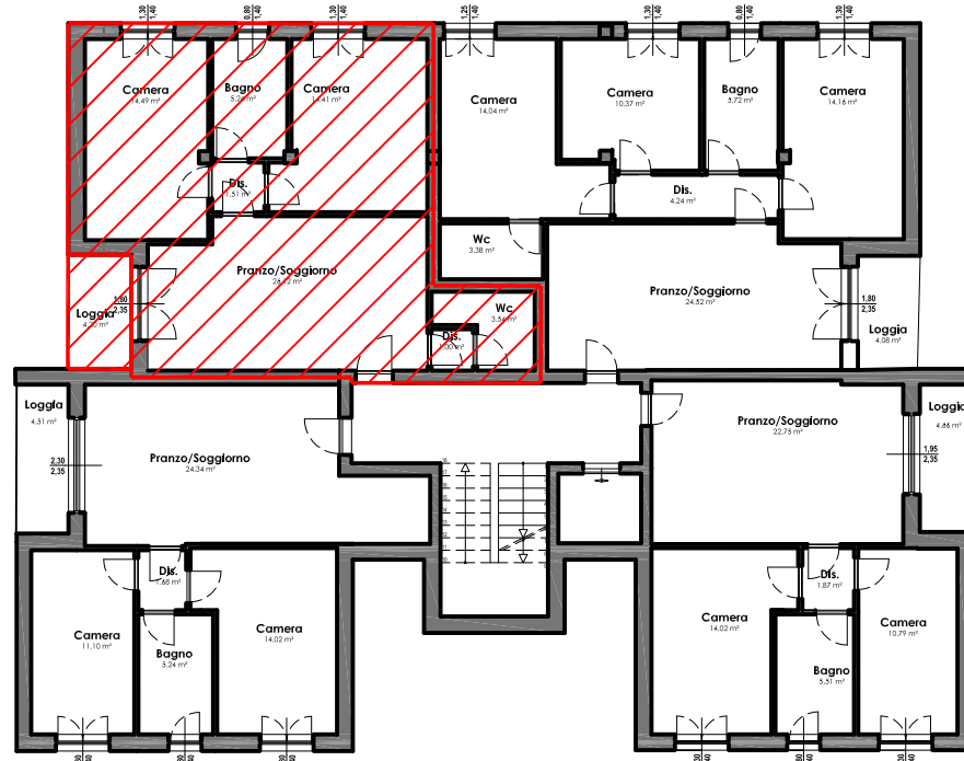
INQUADRAMENTO SCALA 1:200
