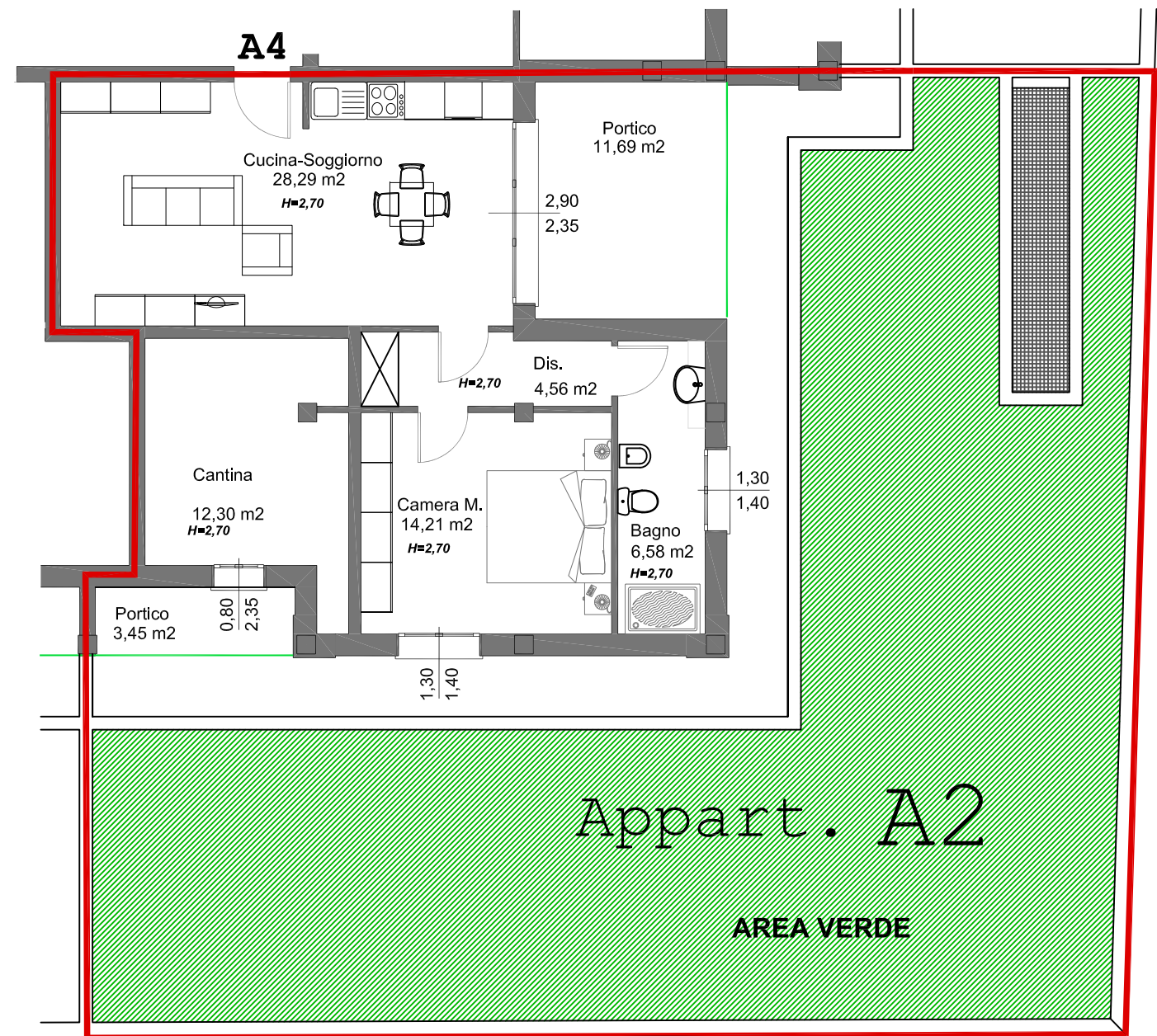
ALLOGGIO SCALA 1:100
