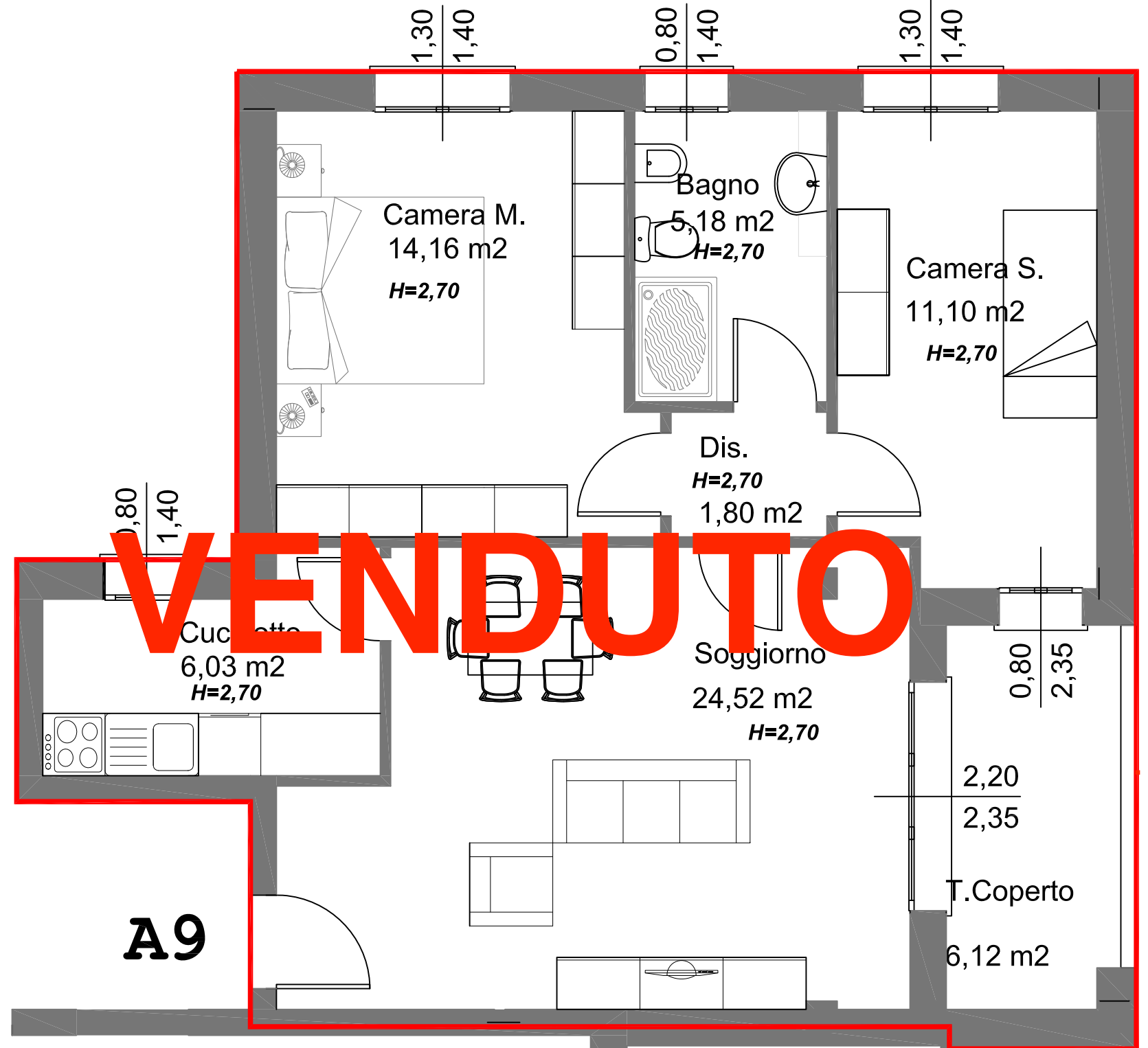
ALLOGGIO SCALA 1:50
