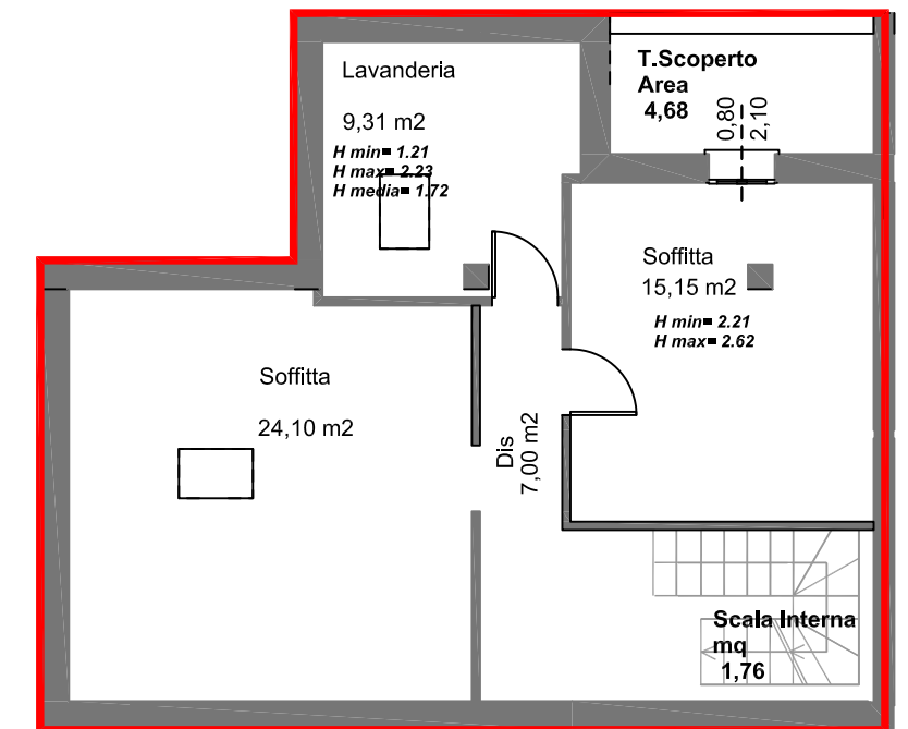
ALLOGGIO PIANO QUARTO SCALA 1:100
