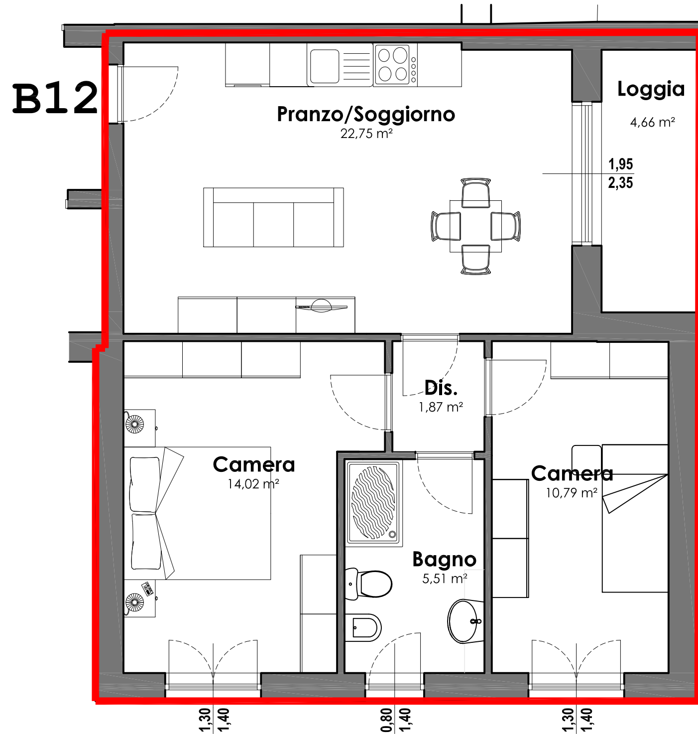
ALLOGGIO SCALA 1:50
