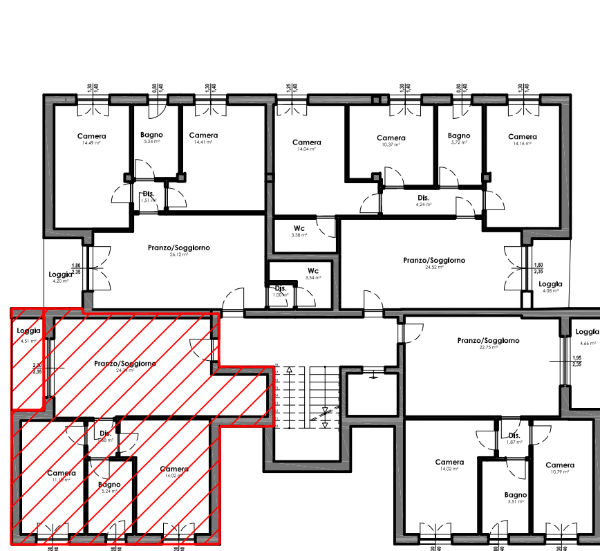
INQUADRAMENTO SCALA 1:200
