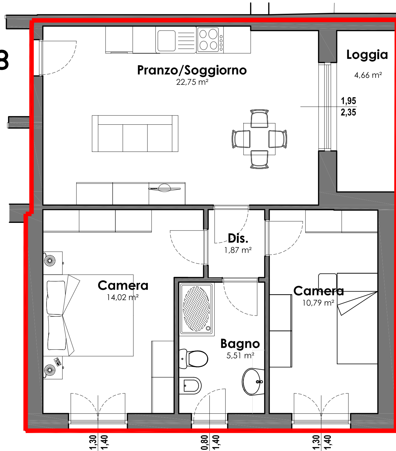
ALLOGGIO SCALA 1:50
