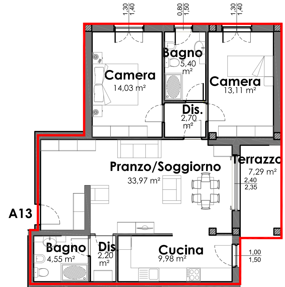
ALLOGGIO SCALA 1:100
