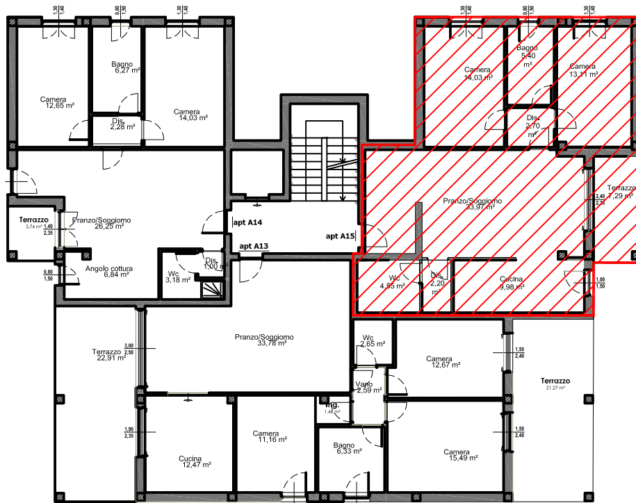
INQUADRAMENTO SCALA 1:200
